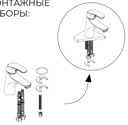
КЛАССИЧЕСКИЙ МОНТАЖНЫЙ НАБОР
